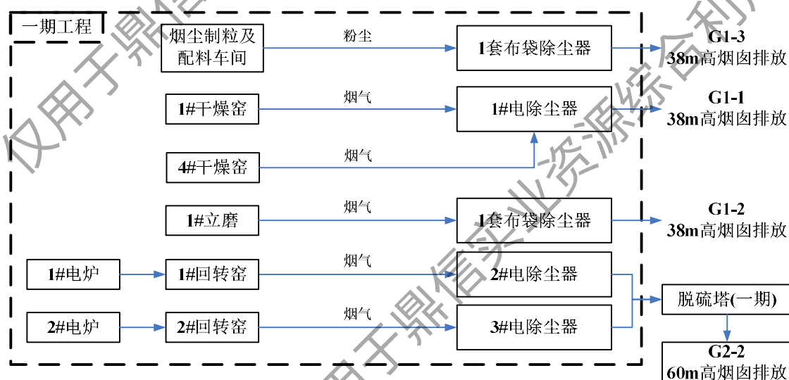
图 3.6-2 技改后一期工程烟气排放示意图
