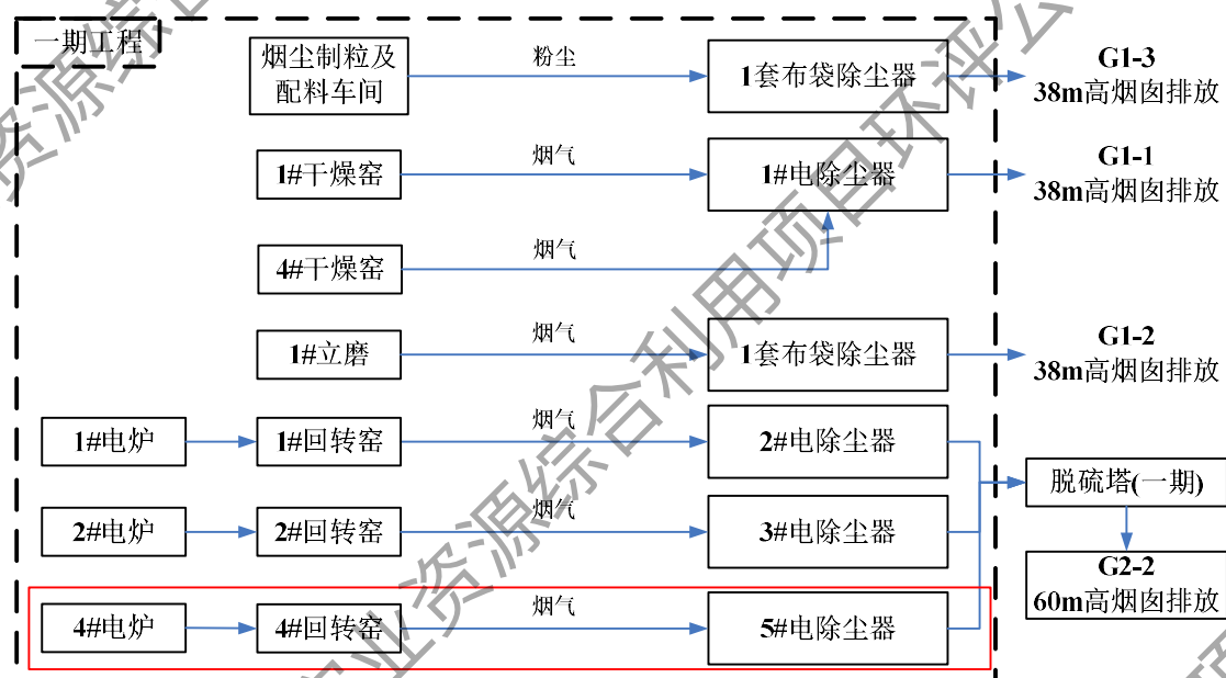
图 3.6-1 技改前一期工程烟气排放示意图
