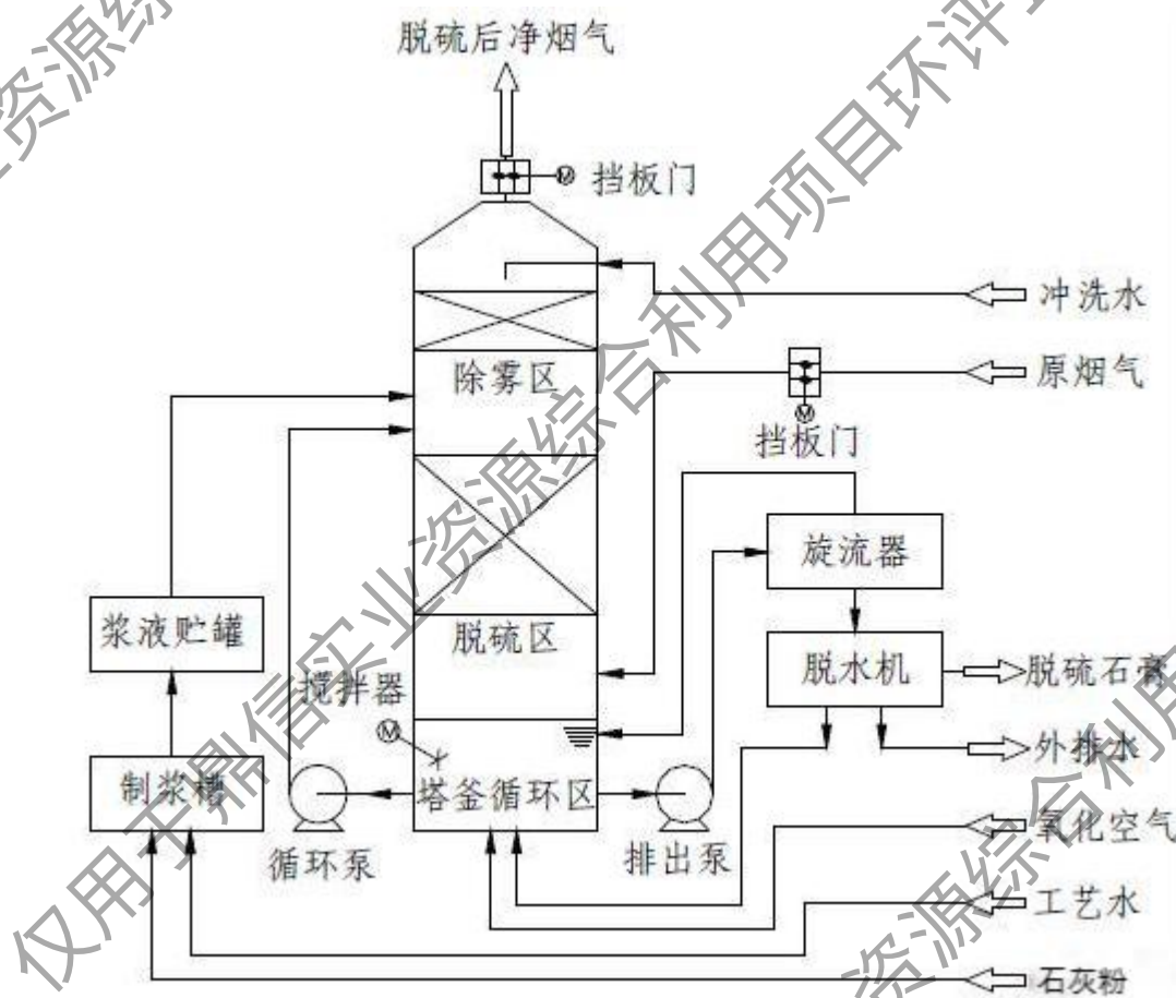
图 7.2-2 石灰石-石膏湿法烟气脱硫工艺流程
